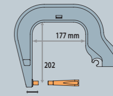
C8 8 bar/550 daN 021440 020016
