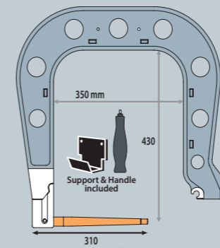
C7 8 bar/550 daN 021433 020009
